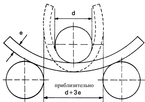
Схема испытания на изгиб
