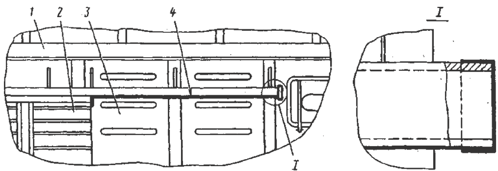
7.5-15 sz. ábra Az oldalfal befedése: 1–tető 2–ajtószárny 3 – oldalfal 4 – üvegszövet
