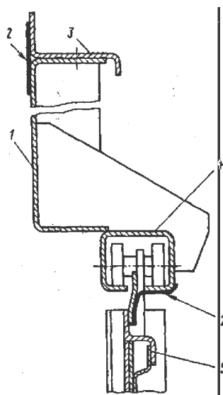
7.5-15 sz. ábra Az oldalfal befedése: 1–tető 2–ajtószárny 3 – oldalfal 4 – üvegszövet
