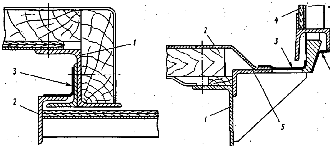
Рис. 7.5-14 Заделка порога дверного проема:
