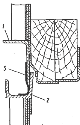
7.5-17 sz. ábra Az oldalfal befedése:
