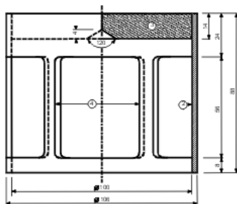
Рис. 2.1. Колоколообразный груз массой 2220 г, который устанавливается на бронзовый поршень
