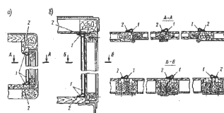
7.5-9 sz. ábra A fa (a) és fém (b) konténer ajtónyílás-hézagainak tömítése nátronpapírral:
