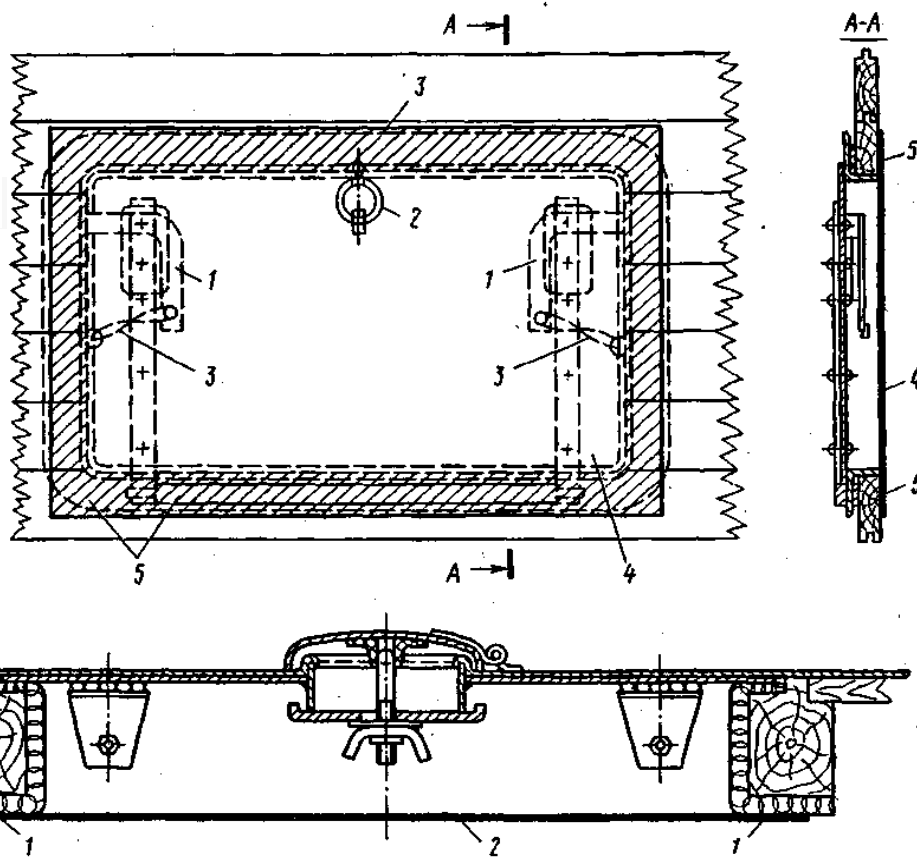
Рис 7.5-2 Заделка печной разделки крафт-бумагой:
