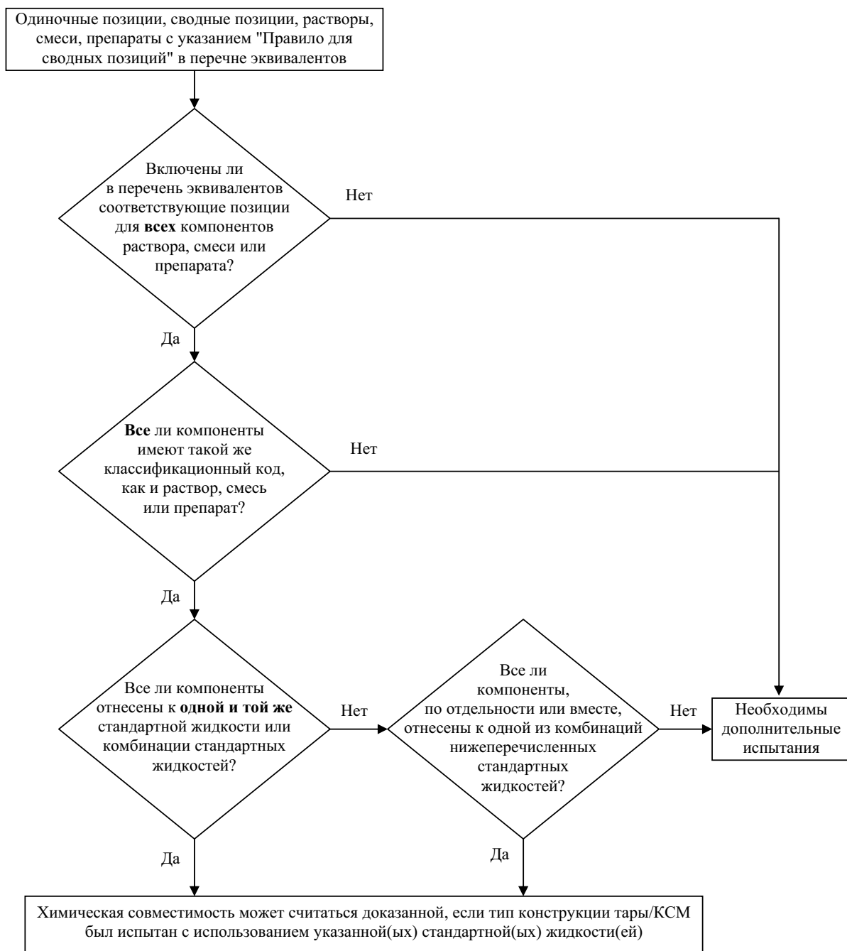
Рисунок 4.1.1.19.2. Блок-схема "Правила для сводных позиций"
