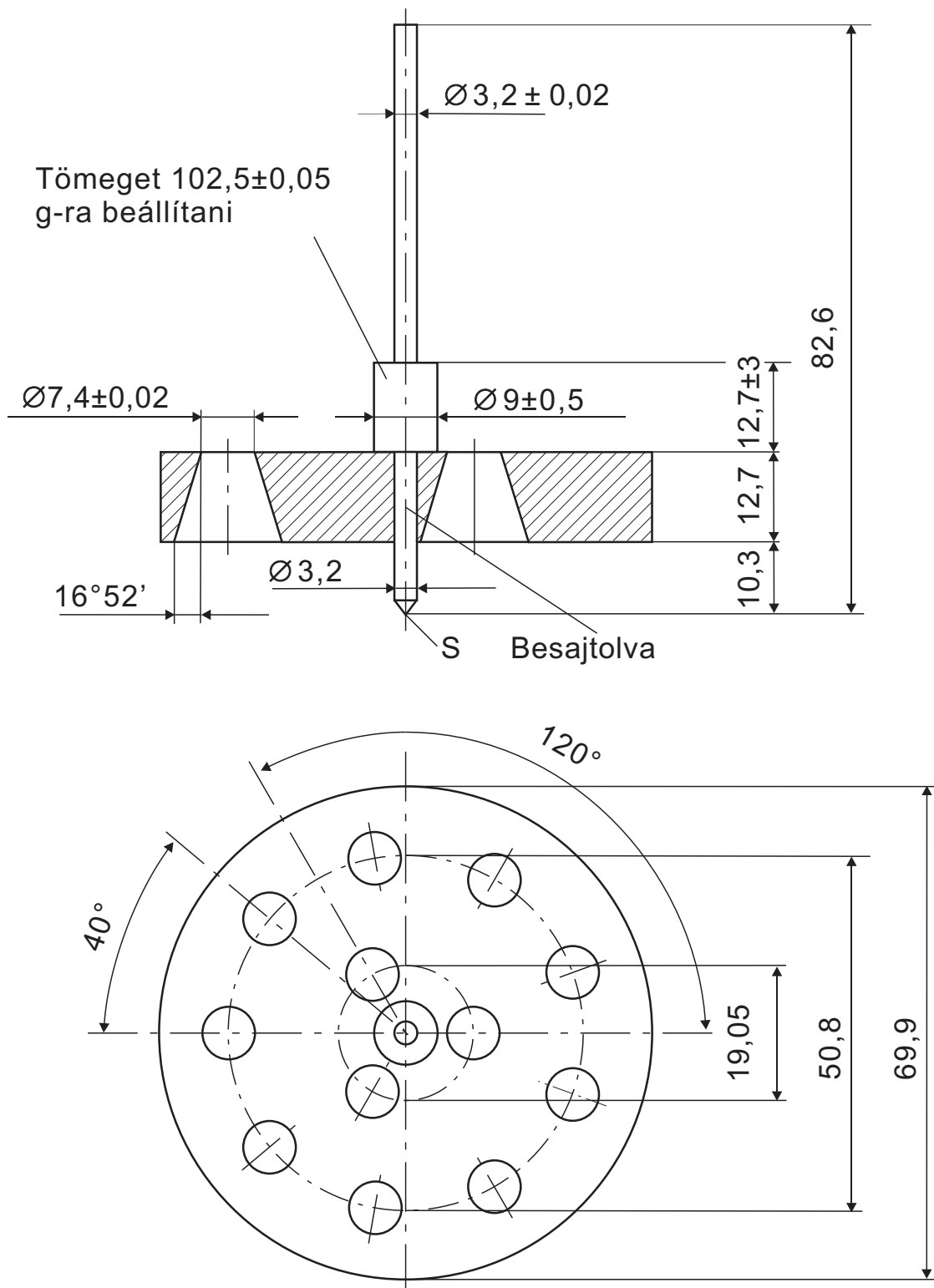
4. ábra: Penetrométer
