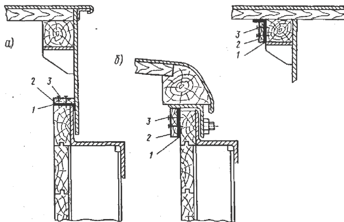
7.5-5 sz. ábra Hézagok tömítése/befedése a tetőszaluzat illesztékeiben a fékező peronra kivezető homlokfal bélelésével:
