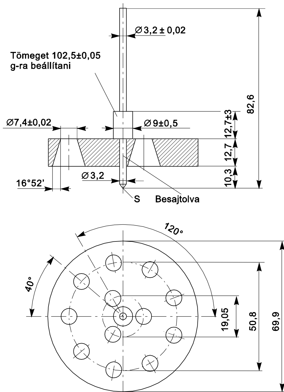
4. ábra: Penetrométer
