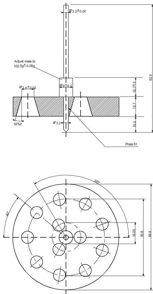
Рис. 2.4. Пенетрометр
