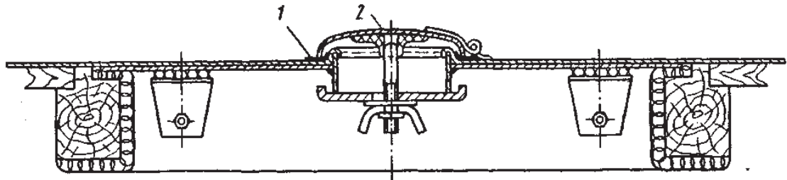
Рис. 7.5 -7 Заделка печной разделки при помощи войлочной прокладки:
