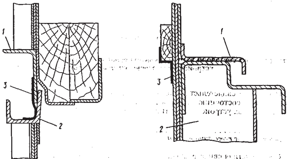
Рис. 7.5-17. Заделка зазора между створками дверей:
