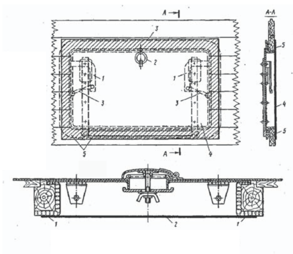
7.5-2 sz. ábra A fűtőnyílás befedése nátronpapírral:
