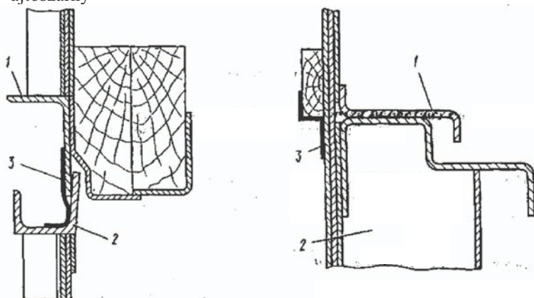
7.5-17 sz. ábra Az oldalfal befedése:
