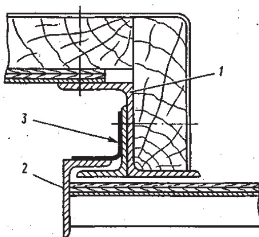
Рис. 7.5-13 Заделка дверного проема:
