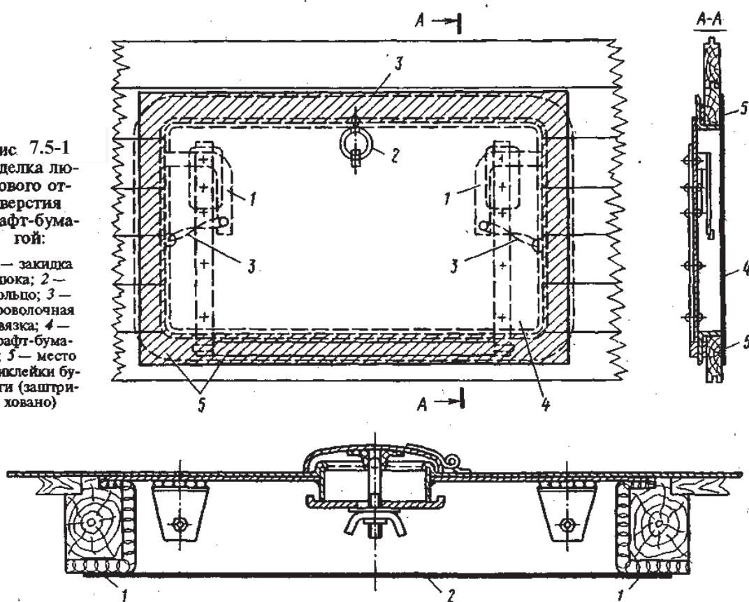
Рис 7.5-2 Заделка печной разделки крафт-бумагой:
