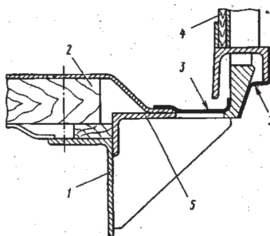
Рис. 7.5-14 Заделка порога дверного проема:
