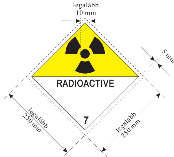
7D sz. nagybárca a 7 osztály radioaktív anyagaihoz
