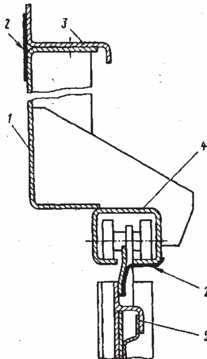
Рис. 7.5-16. Заделка верхней части дверного проема:
