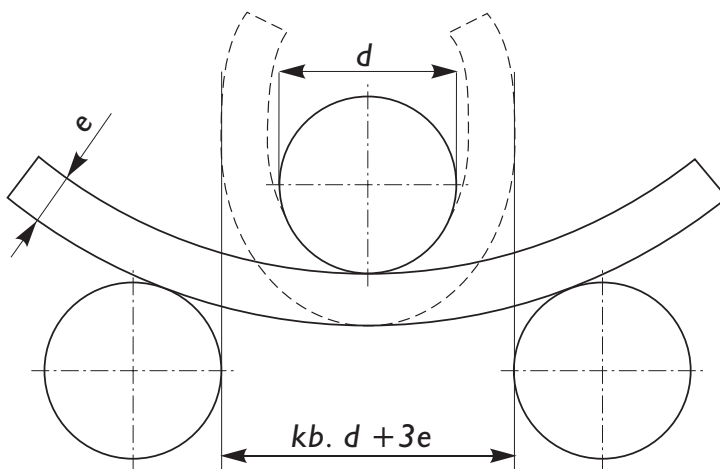
A hajlítási próba vázlata
