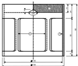
Рис. 2.1. Колоколообразный груз массой 2220 г, который устанавливается на бронзовый поршень, размеры в мм
