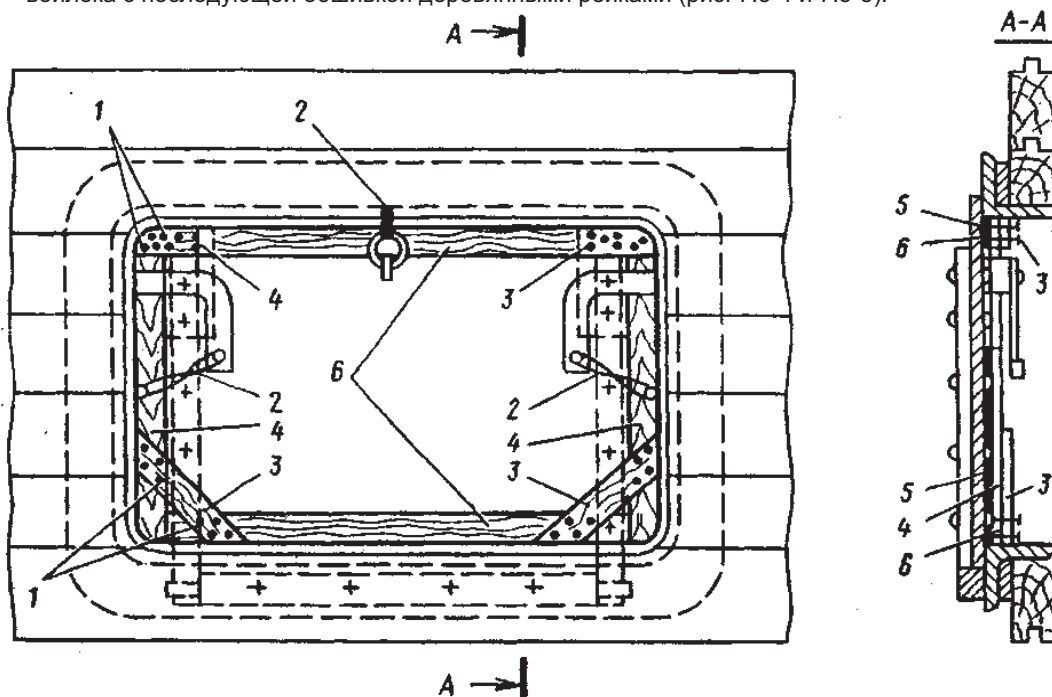
Рис. 7.5-6 Заделка люкового отверстия деревянными планками:
