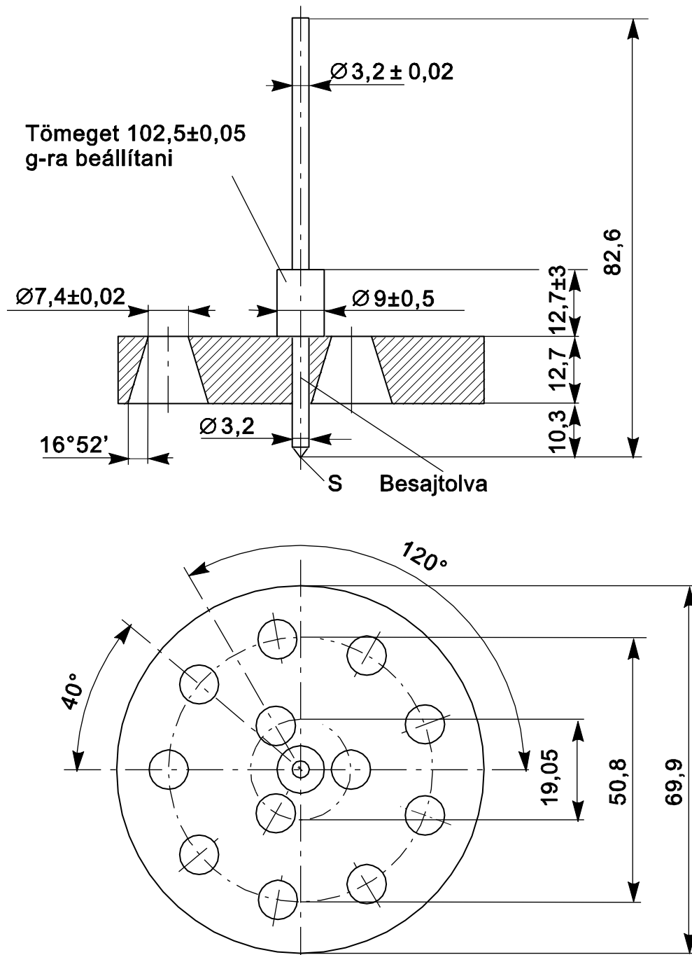
4. ábra: Penetrométer
