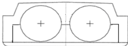
N típus 2.,3. vagy 4. rakománytartály-konstrukció
