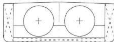
C típus 1. rakománytartály-konstrukció
