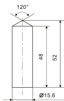
2. ábra: Hengeres bronzdugattyú, méretek mm-ben
